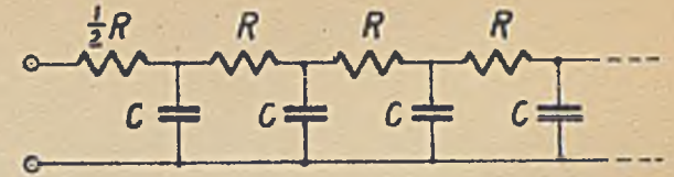
Rys. 24. Przykład linii sztucznej.
