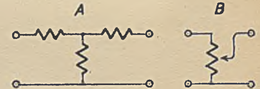
Rys. 25. Przykłady tłumików.
