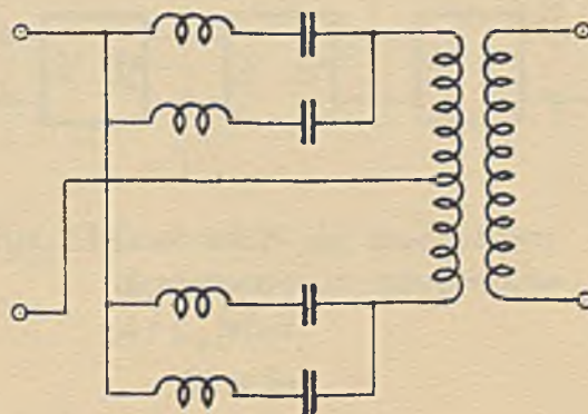
Rys. 17. Przykład filtra różnicowego.
