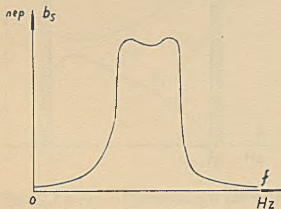
Rys. 14. Tłumienie skuteczne filtra pasmowozaporowego (przykład).
