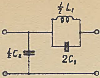
Rys. 20. Ogniw równoległe-pochodne ogniwa podstawowego, jak na rys. 18, jeżeli:
