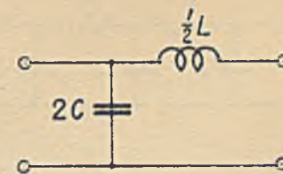
Rys. 18. Przykład ogniwa podstawowego filtra drabinkowego.
