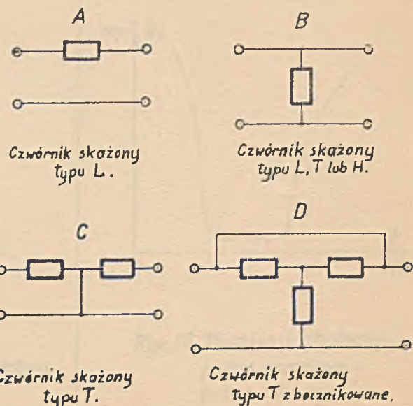
Rys. 7. Czwórnik skażone.
