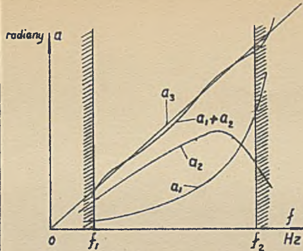
Rys. 22. Korekcja fazowa w zakresie częstotliwości od f_1 do f_2 .
