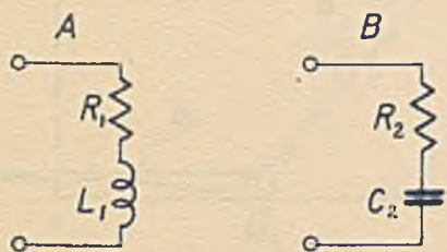
Rys. 5. Dwojniki A i B są sprzężone dla częstotliwości f = \frac{1}{2\pi\sqrt{L_1 C_2}} , gdy R_1 = R_2 .
