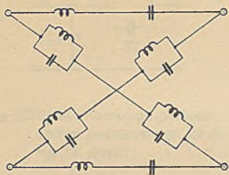
Rys. 16. Przykład filtra krańcowego.
