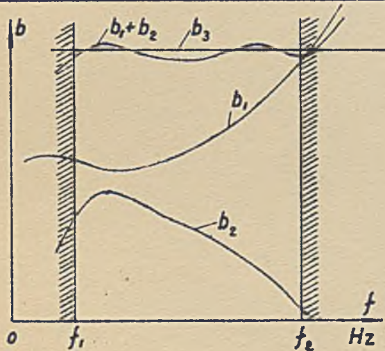
Rys. 21. Korekcja tłumieniowa w zakresie częstotliwości od f_1 do f_2 .
