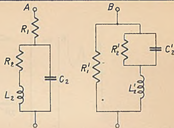
Rys. 4. Dwojniki A i B są przeciwstawne,
