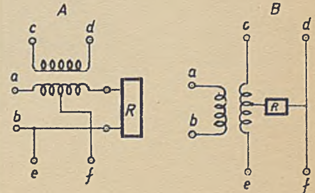
Rys. 26. Przykłady rozgałęźników. R - równoważnik.
