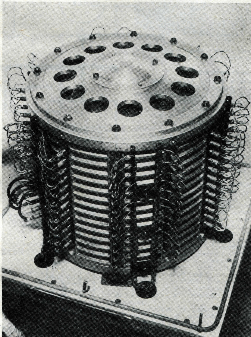
Bęben magnetyczny urządzenia pamięci maszyn rodziny ZAM
