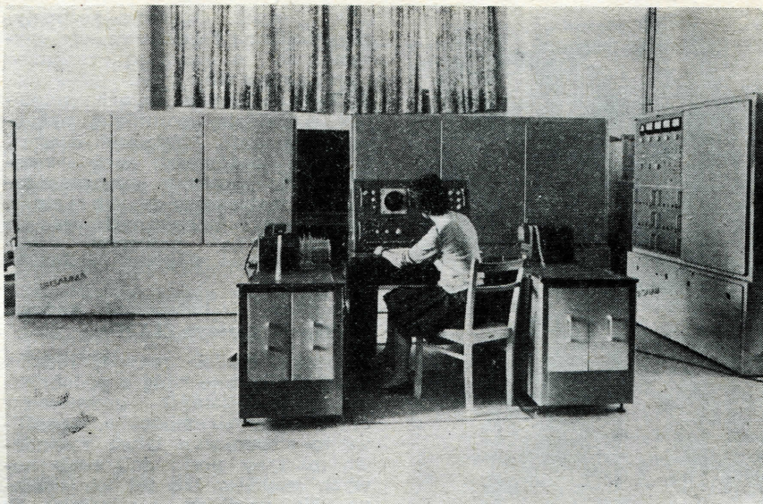
Mała cyfrowa maszyna matematyczna ZAM-2 Gamma
