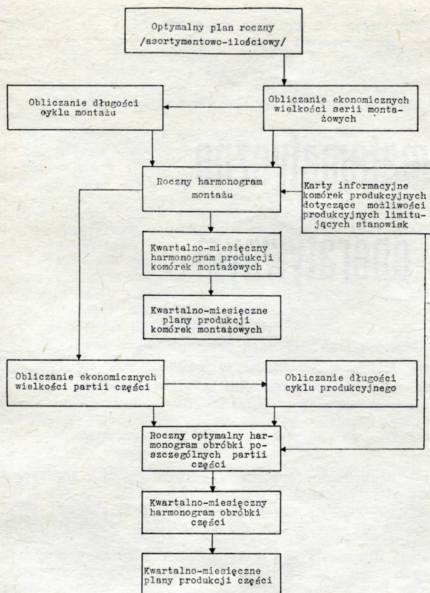
Rys. 1. Przebieg planowania operatywnego
