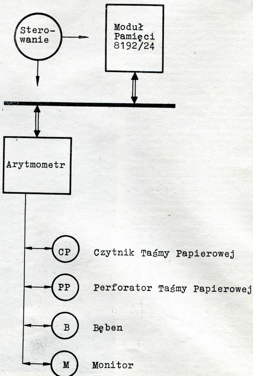
Rys. 1. Zestaw maszyny ZAM-11 lub ZAM-21 do obliczeń naukowo-technicznych
