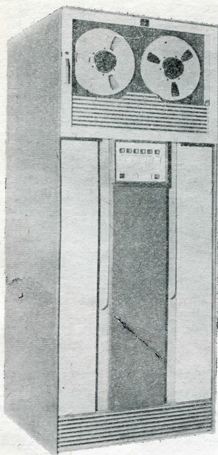
Stacja magnetycznej pamięci taśmowej maszyn rodziny ZAM
