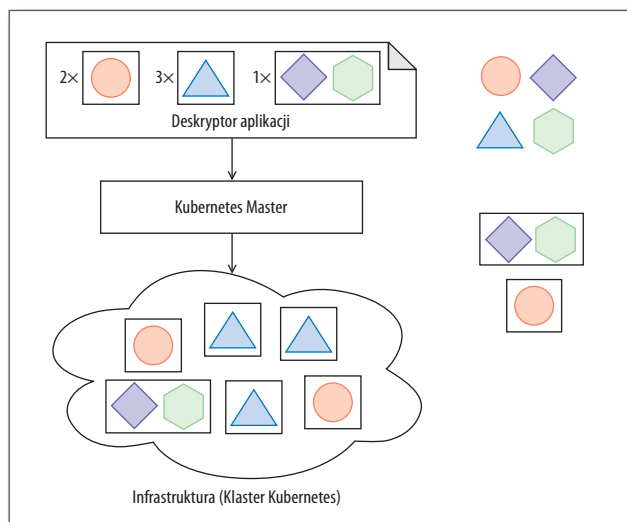
Rys. 1. Idea działania Kubernetes
