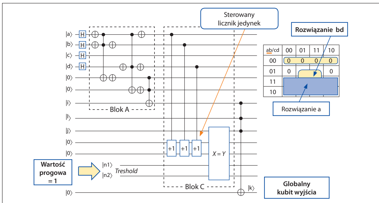
Rys. 3. Pierwsza wyrocznia w sekwencji wyroczni dla rozwiązania problemu minimalnych zbiorów suportujących dla funkcji binarnej z rys. 1 z minimalnym zbiorem zmiennych suportujących \{a, b, d\} . KPN = (a+b) \cdot (a+d) = 1 \oplus (a'b)' \cdot (a'd)' jest realizowana w bloku A. Bramki Hadamarda u góry z lewej nie należą do wyroczni. Bramki te zostały tu umieszczone dla celów dydaktycznych, ponieważ służą one jako generator wszystkich podzbiorów zbioru \{a, b, c, d\} poprzez stworzenie superpozycji wszystkich liczb od 0 do 15. Ta pierwsza wyrocznia weryfikuje, czy istnieje rozwiązanie z kosztem 1, ponieważ wartość ograniczenia Threshold została ustawiona na 1. Tablica Karnaugh pokazuje funkcję (a+b) \cdot (a+d) opisaną przez 0 w kratkach tablicy. Grupa a, która jest pierwszym rozwiązaniem, ilustruje jak wszystkie rozwiązania zawarte w a są następnie zastępowane przez 0. Po tym zastąpieniu pozostaje jedynie iloczyn logiczny bd(a)' .
