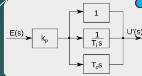
Schemat idealnego regulatora PID, zawierającego bloki Proporcjonalny(P), Całkujący(I) i Różniczkujący(D)
