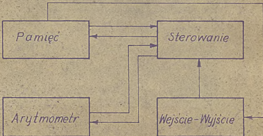
Rys.1. Schemat blokowy przebieżnikowej maszyny cyfrowej.
