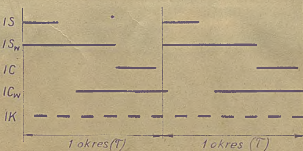
Rys. 6. Impulsy nadajnika w skali czasowej.
