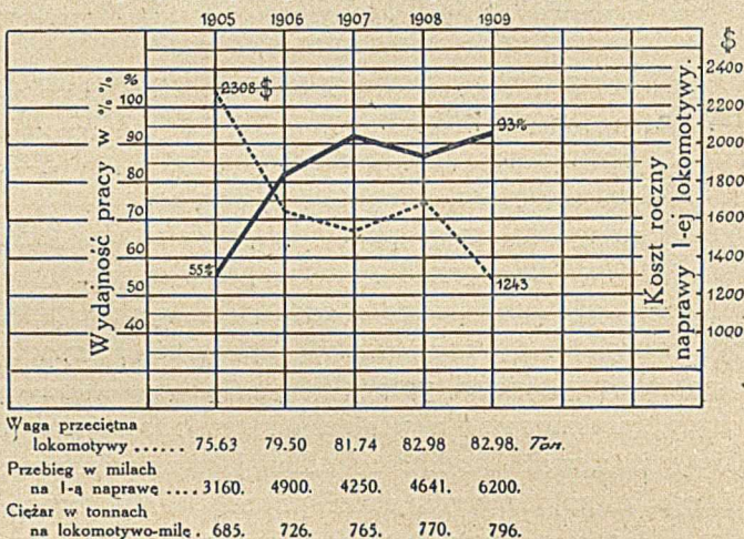
Fig. 1. Wydajność pracy i koszt naprawy lokomotyw.
