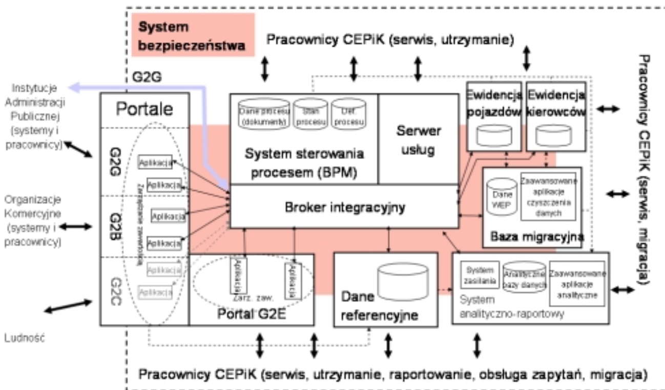
Diagram 3 Ogólna koncepcja architektury systemu.
