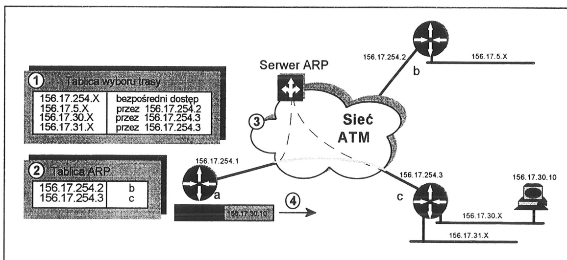
Rys. 3. Wybór trasy pakietów IP w sieci ATM.
