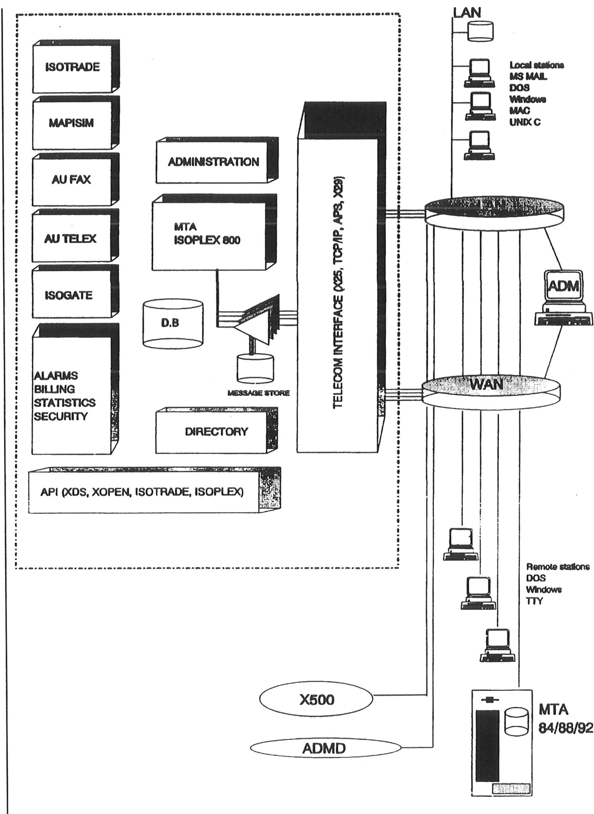
Rys. 2. : Struktura funkcjonalna systemu POLKOM/400
