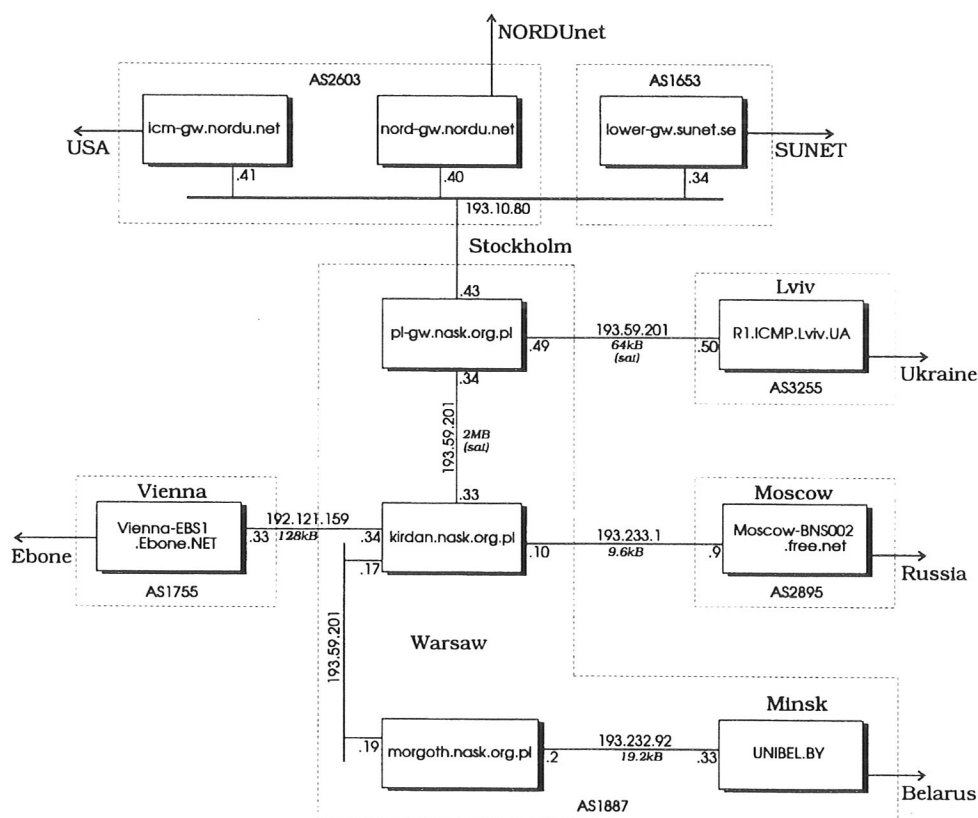
Połączenia międzynarodowe z NASK
