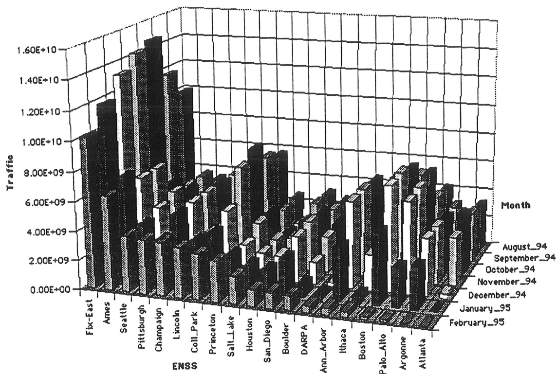
Rys. 3. Statystyki ruchu na różnych liniach dostępowych do szkieletu sieci NSFnet przeprowadzone w okresie lipiec 1994 - luty 1995. Rysunek obrazuje proces stopniowego wyłączania sieci NSFnet.
