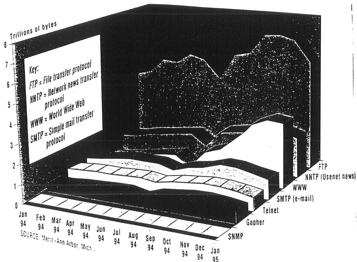
Rys. 2. Statystyka ruchu w szkieletcie sieci NSFnet w okresie styczeń 1994 r. - styczeń 1995 r. Dominująca aplikacja jest FTP. Od połowy 1994 r. Następuje gwałtowny wzrost transmisji WWW. Minimum w połowie 1994 r. jest spowodowane okresem wakacyjnym. Końcowe minimum jest związane ze stopniowym wyłączaniem sieci.
