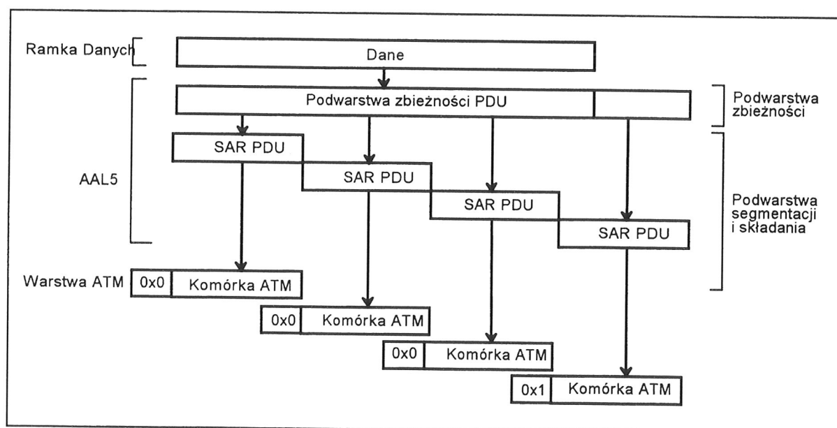
Rys. 2. Sposób upakowania pakietów protokołów warstw wyższych w komórkach ATM
