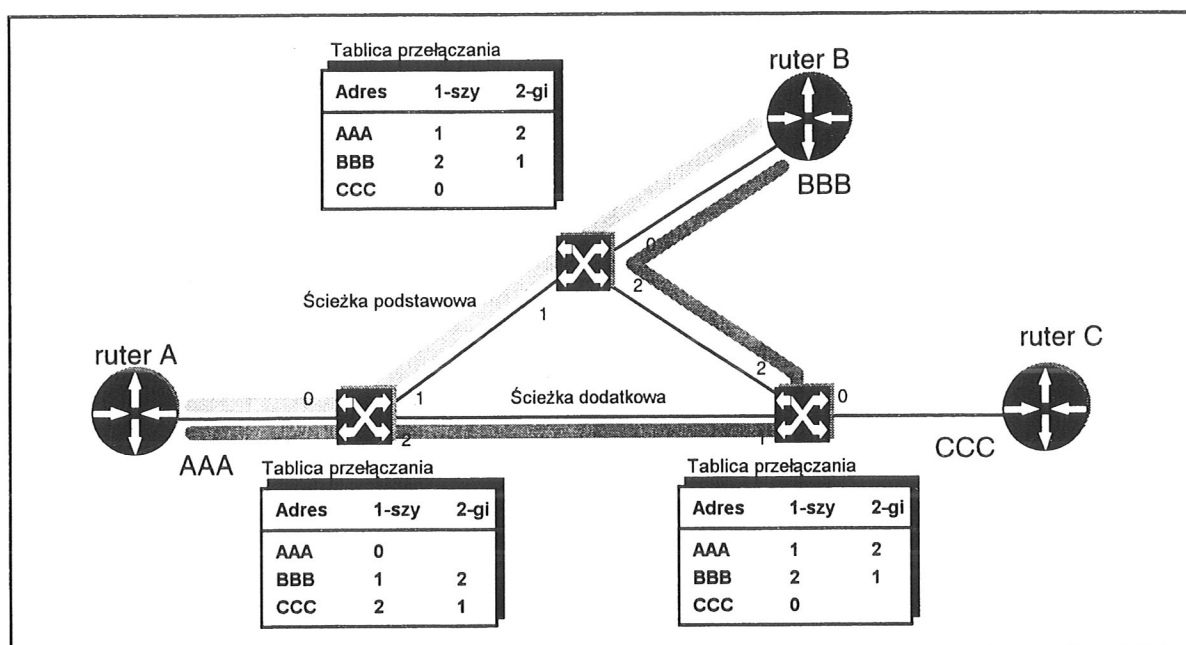
Rys. 5. Realizacja alternatywnego połączenia wirtualnego z wykorzystaniem SVC
