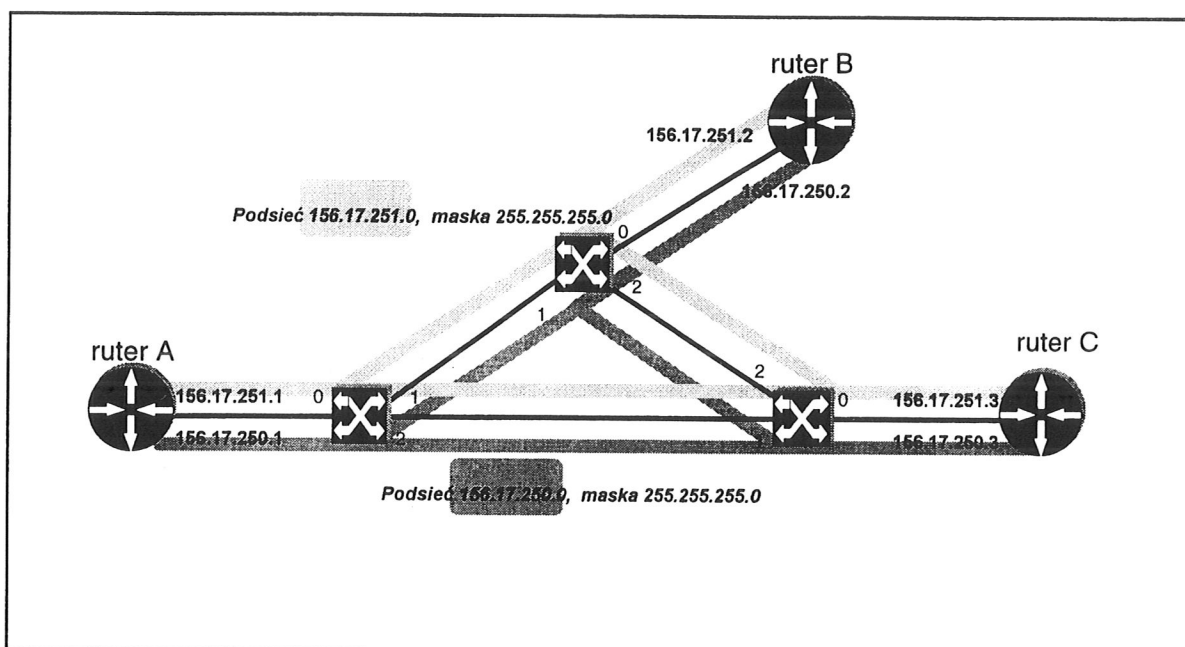
Rys. 4. Dwie podsieci IP realizowane na dedykowanych PVC.
