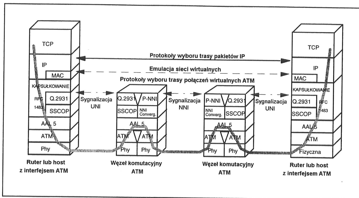
Rys. 1. Model transmisji IP przez sieć ATM
